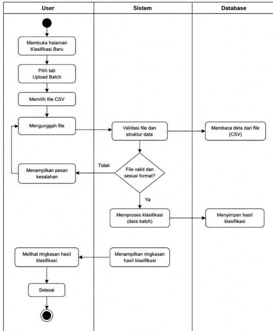
Gambar 3.6 Activity Diagram Klasifikasi Batch
