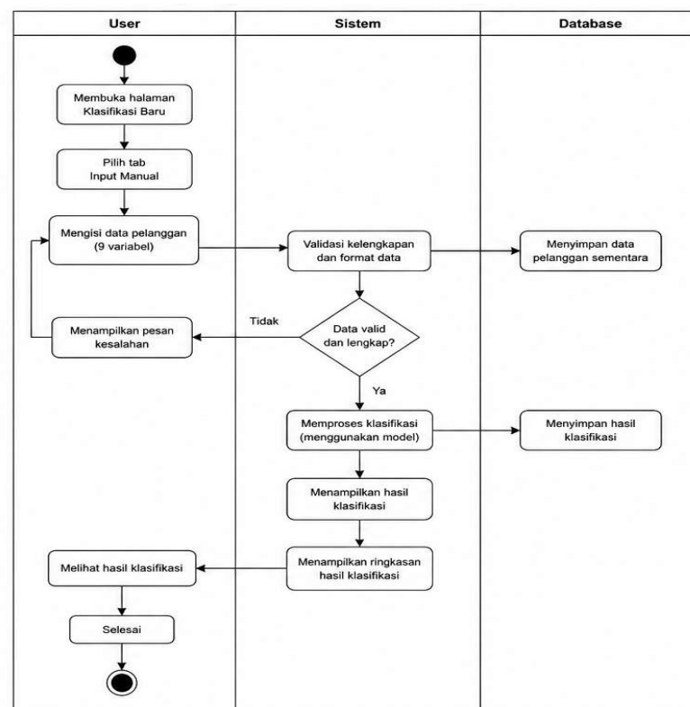
Gambar 3.5 Activity Diagram Klasifikasi Manual
